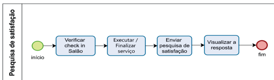
Figura 2. Processo Pesquisa de Satisfação.
